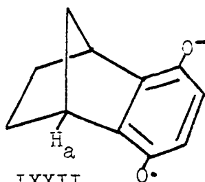
LXXII a_{H_a}^H < 0.1
