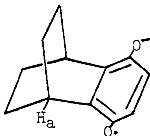
LIV a_{H_a}^H < 0.1
